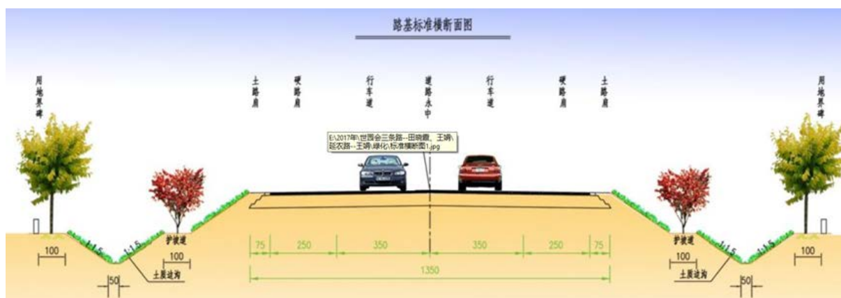
图 2-1 本项目环评阶段横断面布置图
