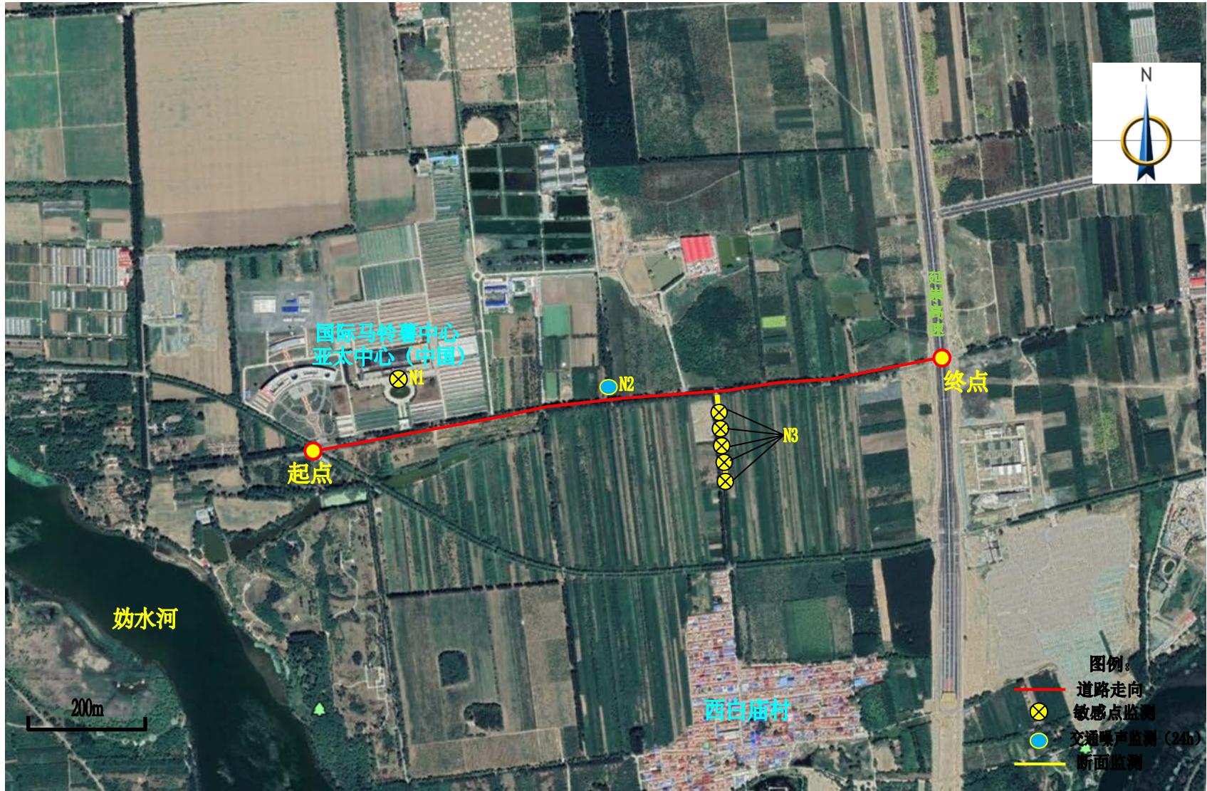
图 6-1 噪声监测点位图
