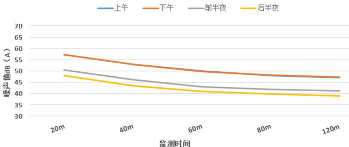
图 6-3 衰减断面噪声随距离变化图 (N3)
