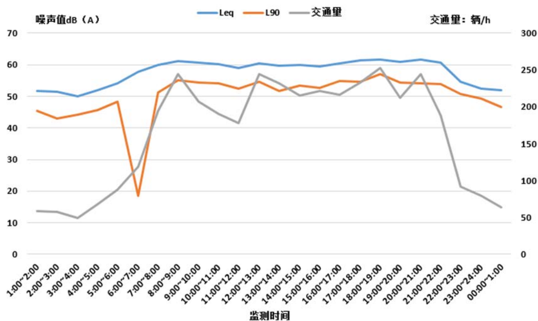
图 6-2 24h 交通噪声监测结果图
